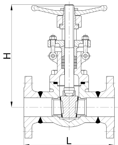
ZZK16.k / ZZK25.k / ZZK40.k
