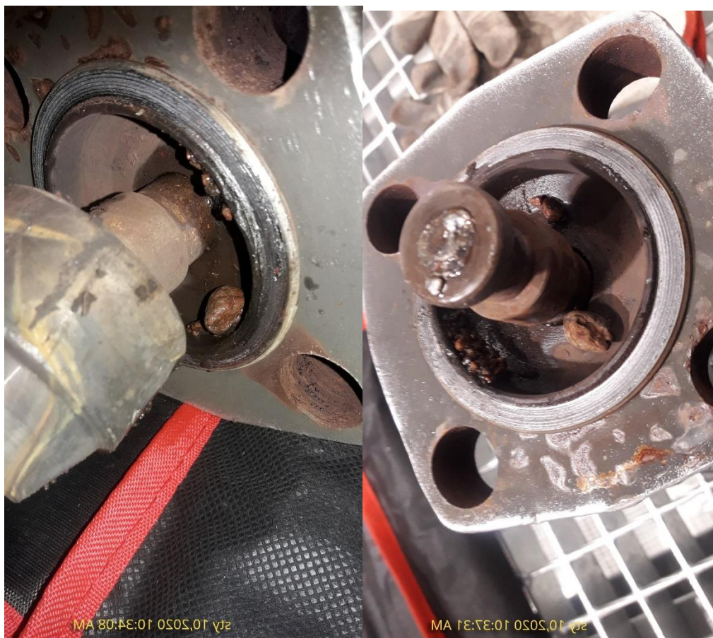
Kamienie w korpusach zaworów (prawdopodobnie dostały się do korpusów wraz z medium)
