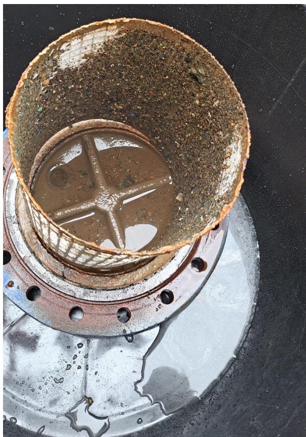
Sito filtra użytego do separacji cząstek stałych na instalacji.
