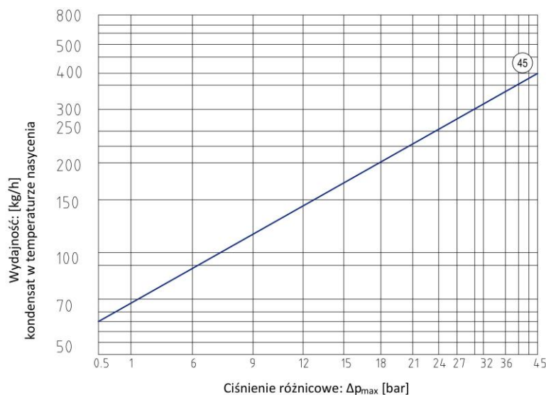
Wykres maksymalnego przepływu kondensatu w zależności od ciśnienia różnicowego.
